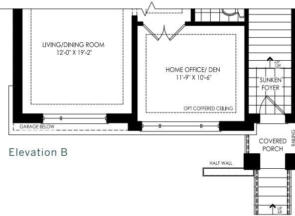
Elevation B
